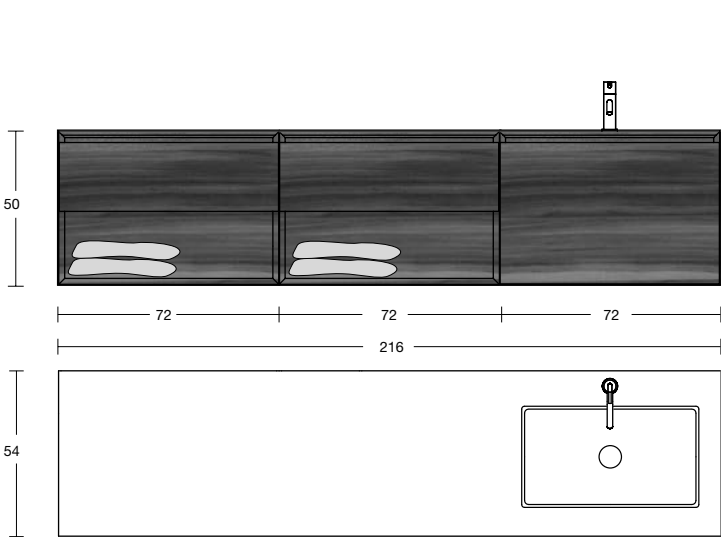
VERSIONE DX - Right version - Version rechts Version droite - Versión derecha - Прав. вариант
