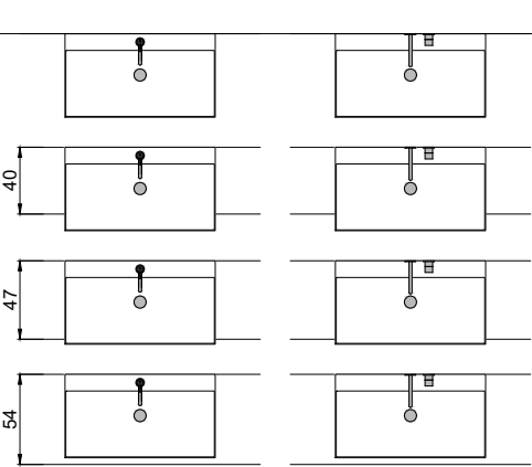
schema d' installazione lavabi e rubinetteria / sinks and taps installation layout
