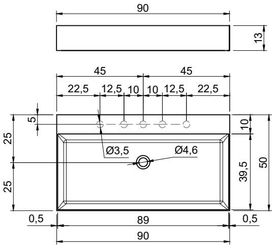
schema d' installazione lavabi e rubinetteria / sinks and taps installation layout
