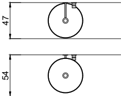
schema d' installazione lavabi e rubinetteria / sinks and taps installation layout
