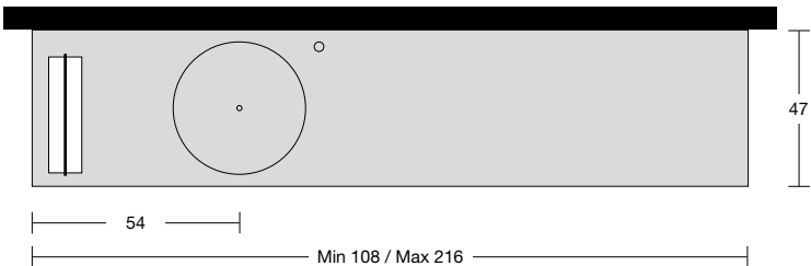
VERSIONE SX - Left version - Version links - Version gauche - Versión izquierda - Лев. вариант
