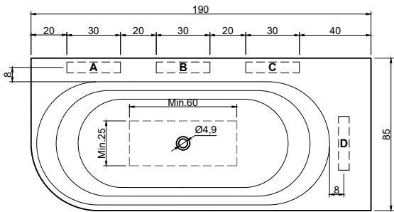
(Vasca decentrata sx o dx ed in basso - versione SX / Off-center bathtub in depth and LH or RH - left version) art. OASI55S peso lordo/gross weight: kg 153 ca peso netto/net weight: kg 128 ca
