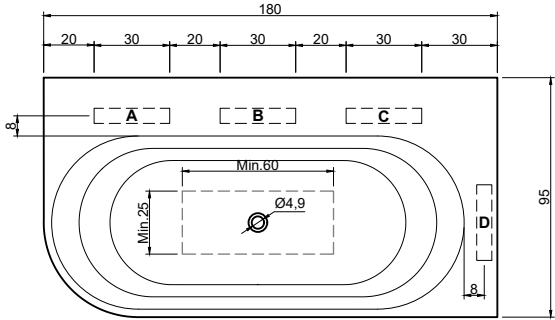
(Vasca decentrata sx o dx ed in basso - versione SX / Off-center bathtub in depth and LH or RH - left version) art. OASI57S peso lordo/gross weight: kg 156 ca peso netto/net weight: kg 131 ca
