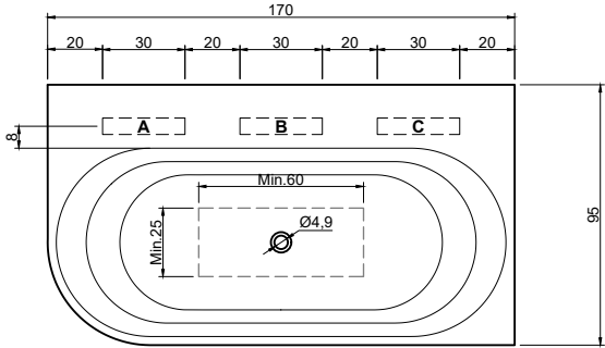
(Vasca decentrata sx o dx ed in basso - versione SX / Off-center bathtub in depth and LH or RH - left version) art. OASI56S peso lordo/gross weight: kg 150 ca peso netto/net weight: kg 125 ca
