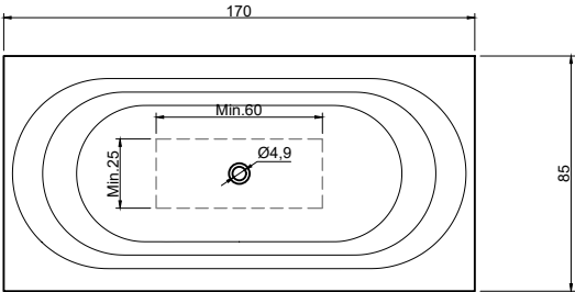
(Vasca centrale / Centered bathtub) art. OASI73M peso lordo/gross weight: kg 204 ca peso netto/net weight: kg 119 ca
