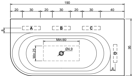
(Vasca decentrata sx o dx ed in basso - versione SX / Off-center bathtub in depth and LH or RH - left version) art. OASI58S peso lordo/gross weight: kg 159 ca peso netto/net weight: kg 134 ca
