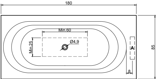
(Vasca decentrata sx o dx - versione sx / Off-center bathtub LH or RH - Left version) art. OASI74MS peso lordo/gross weight: kg 149 ca peso netto/net weight: kg 124 ca
