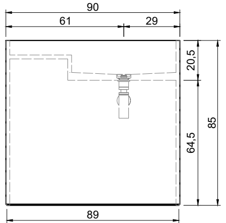
Prospetto frontale Front elevation
