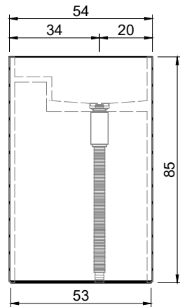
Prospetto frontale Front elevation
