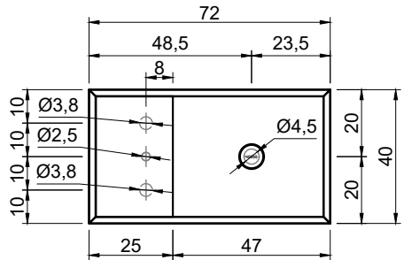
Prospetto frontale Front elevation
