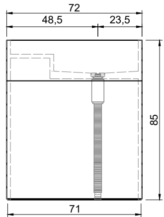
Prospetto frontale Front elevation
