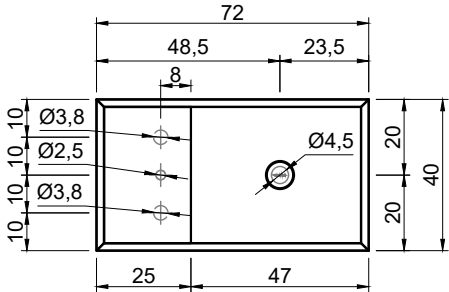
Prospetto frontale Front elevation
