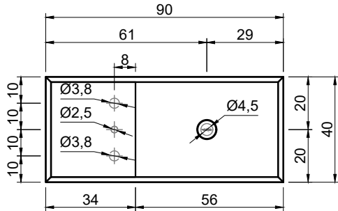
Prospetto frontale Front elevation
