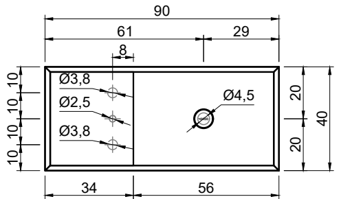
Prospetto frontale Front elevation
