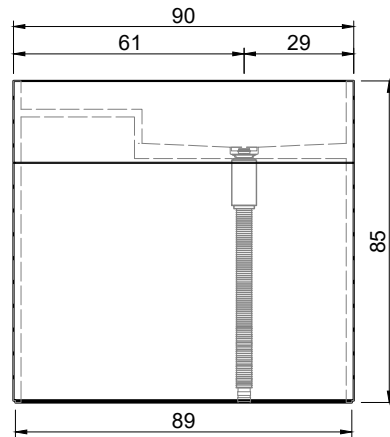
Prospetto frontale Front elevation
